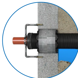
Wanddurchführung
